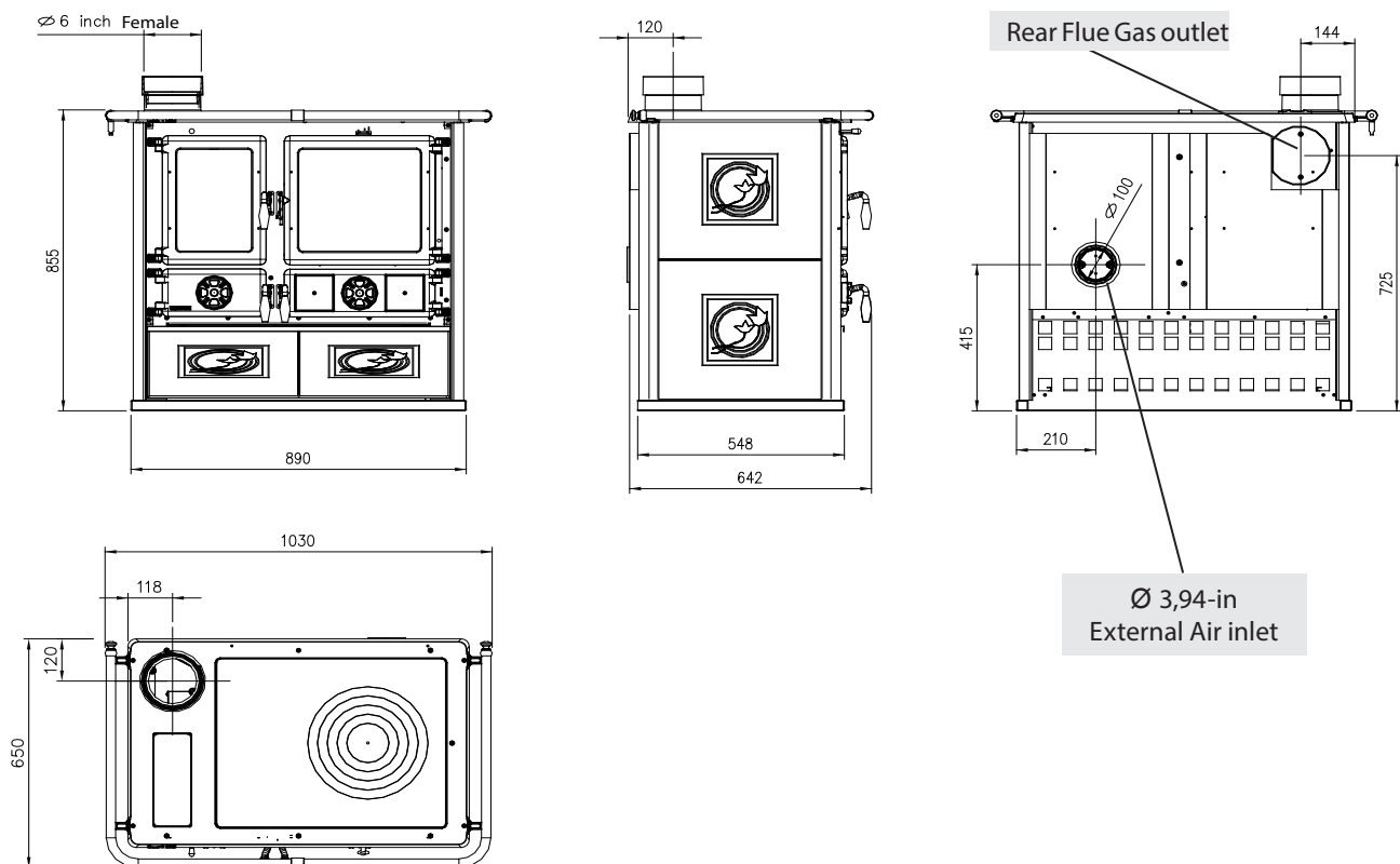
ROSA SINISTRA REVERSE UL-C - 183 kg
