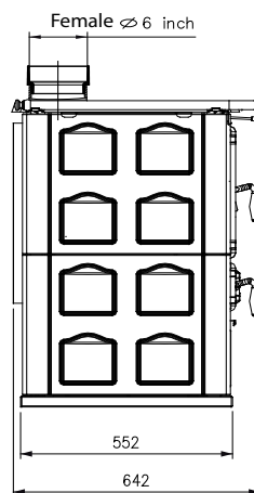
ROSA UL-C - Liberty 183 kg - Petra 200 kg
