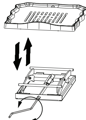
Grille plate de grosse épaisseur réglable en hauteur
